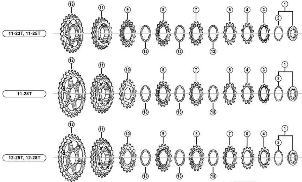
CS-9000 sprocket teeth combinations
